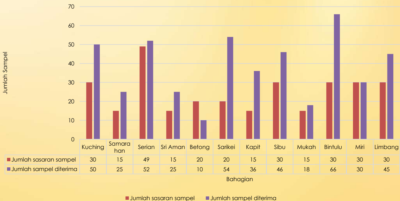
Jumlah Sasaran Sampel yang Diambil bagi Pengujian Penyakit African Swine Fever (ASF) - Babi Domestik/Babi Kampung
